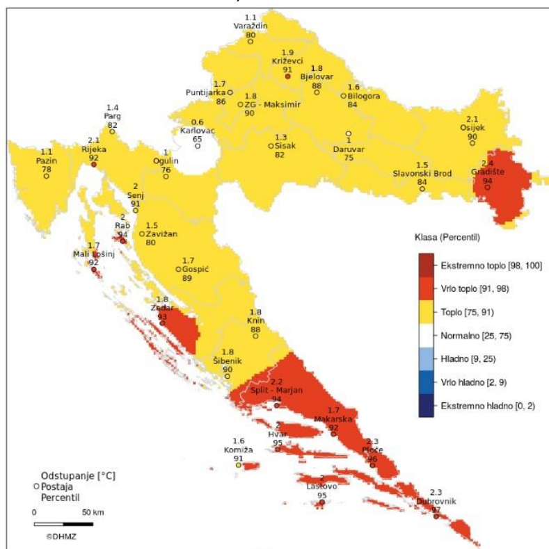
Slika 2. Odstupanje srednje temperature zraka za rujun 2020. godinu za Republiku Hrvatsku
