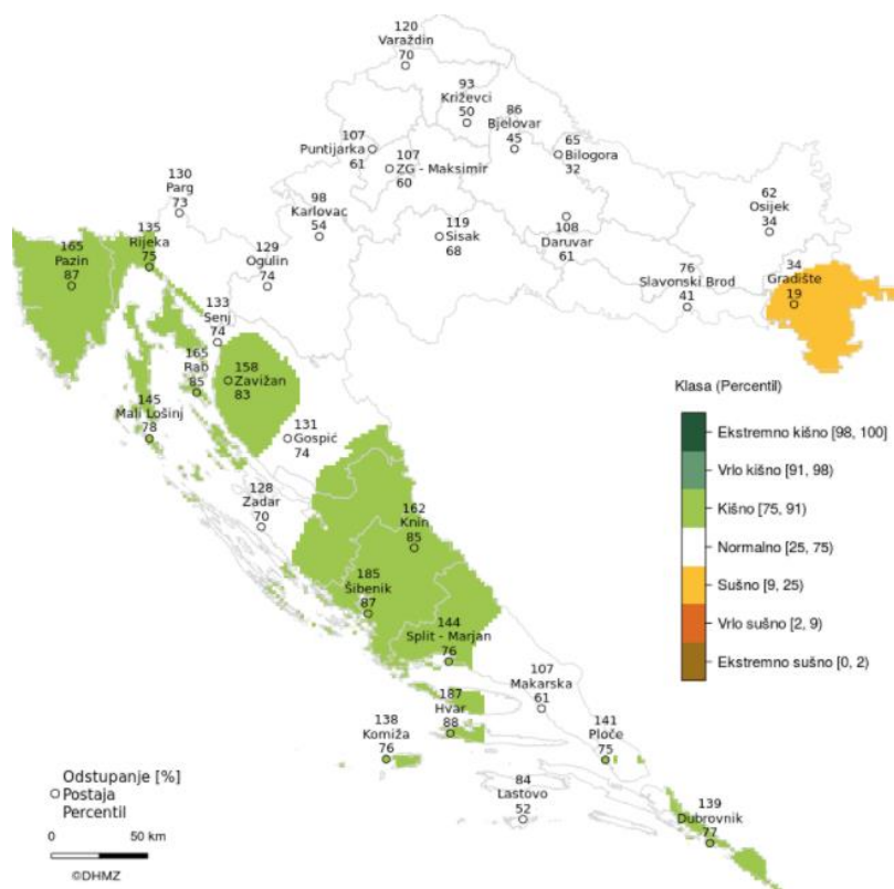
Slika 5. Oborinske prilike u Hrvatskoj za rujan 2020. godine Izvor: DHMZ
